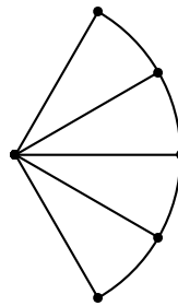
Figure 4: The fan F_5
