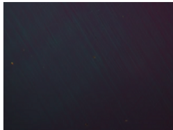
Cubic austenite
